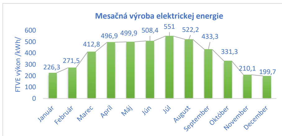
Graf priemernej ročnej produkcie elektrickej energie z fotovoltickej elektrárne
